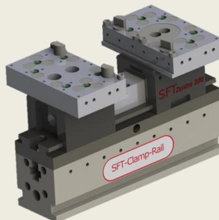
Zentro 300 mit Spannschiene CP300.80.001 Flex-Spannbacken und 2 Stück Spannbacken mit Krallen
