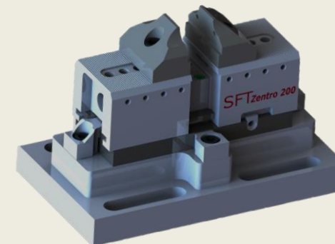
Zentro 200 mit kundenspezifischen Unterbau und 2 Stück M16.3903.03 Zentrobacke oben 30 mm breit mit Krallen
