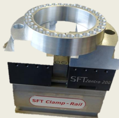
Zentro 200 mit Spannschiene CP200.80.001 und M16.4101.03 Rohbacke Alu
