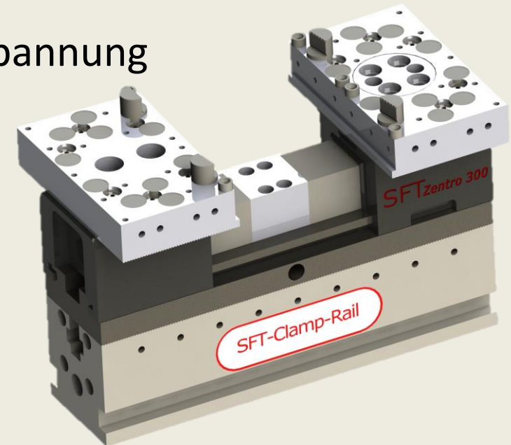
Abbildung Zentro 300 mit Spannschiene CP300.80.001 und Flex-Spannbacken
