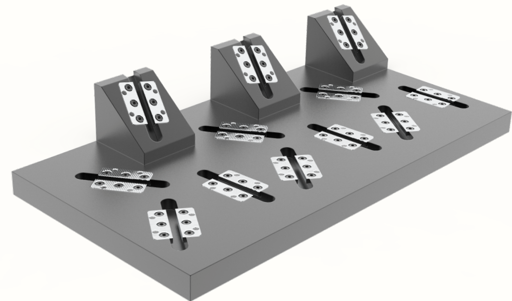
Serienvorrichtung für Schweisskonstruktion series device for welded construction
